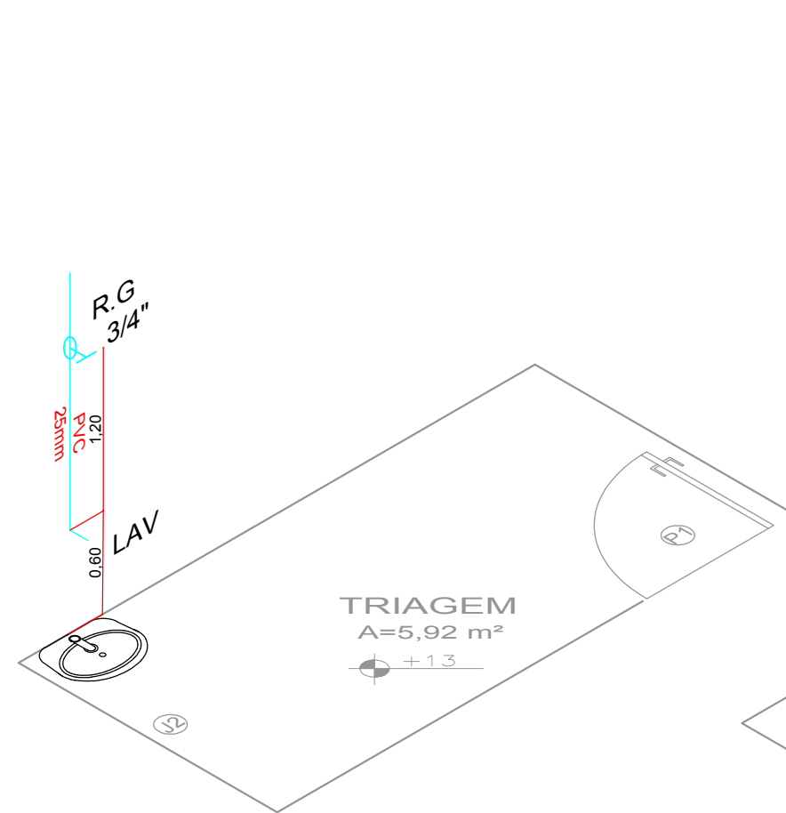
ISOMÉTRICO Triagem Sem Escala
