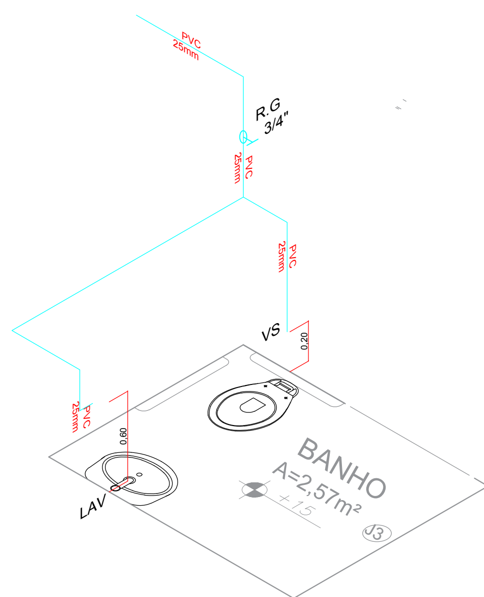
ISOMÉTRICO Banho Sem Escala
