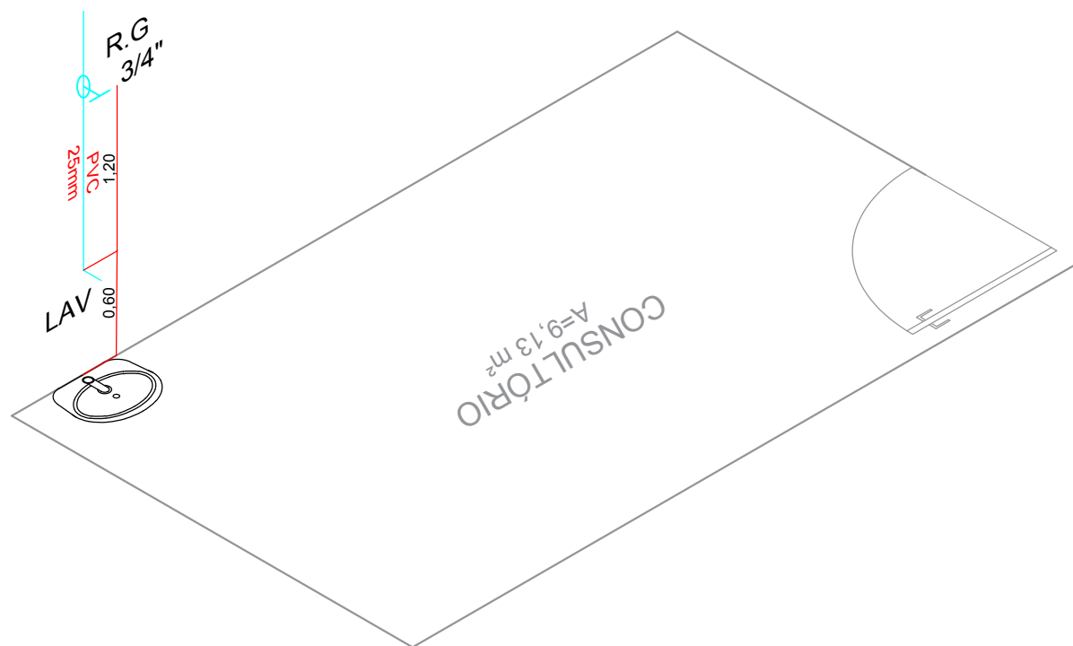
ISOMÉTRICO Consultório Sem Escala
