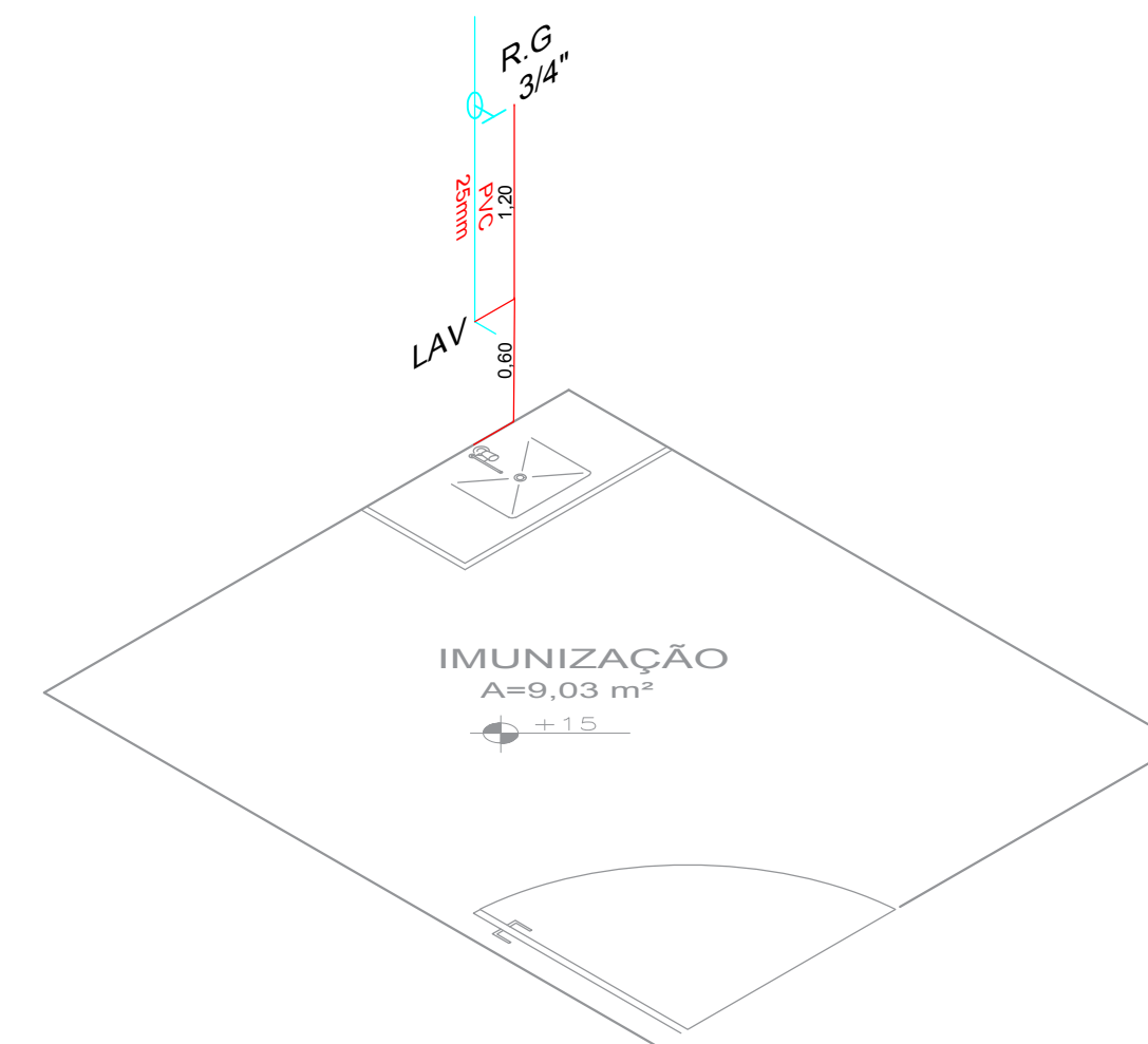
ISOMÉTRICO Imunização Sem Escala
