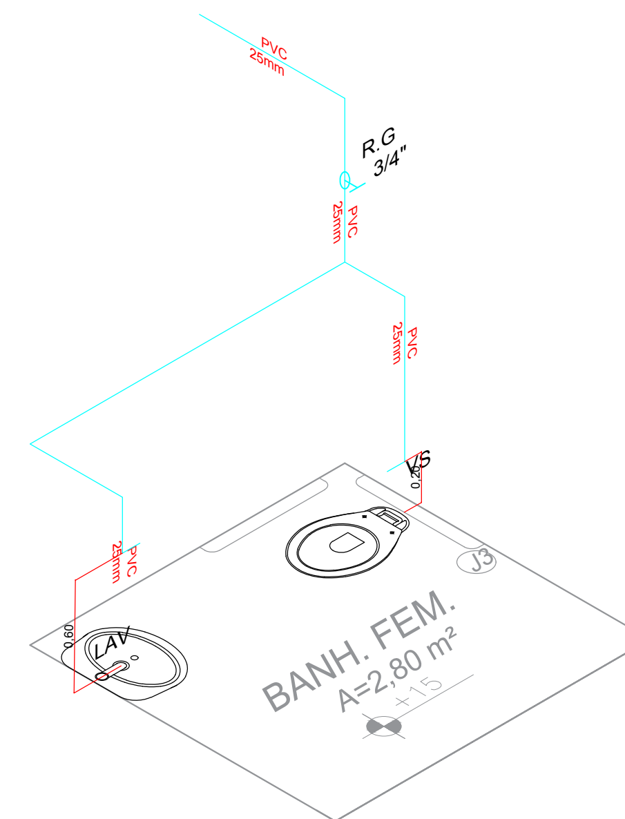
ISOMÉTRICO Banho Fem. Sem Escala
