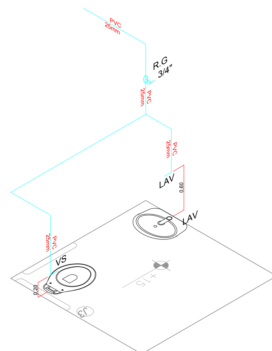
ISOMÉTRICO Banho Masc. Sem Escala
