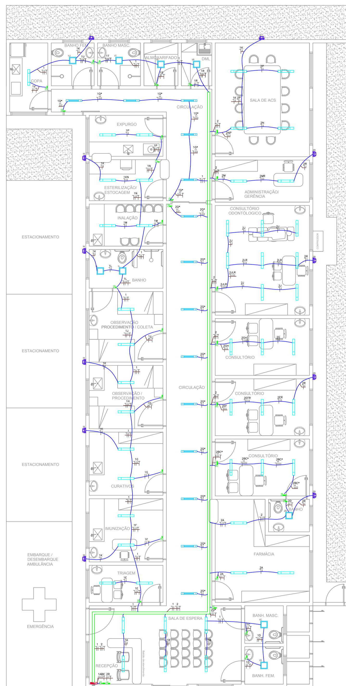
PLANTA BAIXA - ILUMINAÇÃO ESCALA: 1/75
